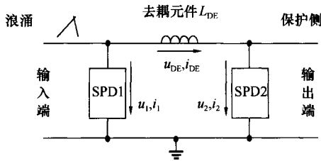
图 13 SPD 能量配合电路模型
